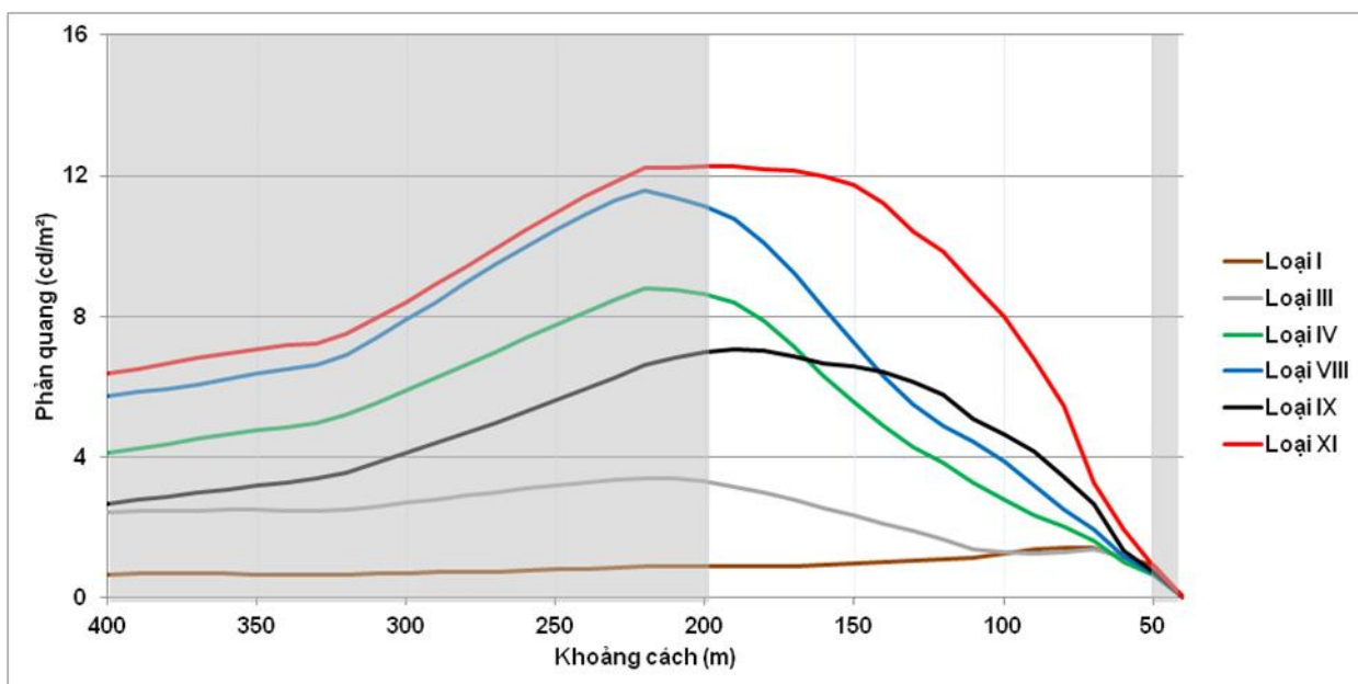
Hình E.6: Độ phản quang cầu biển báo đặt trên giá long môn đối với xe tải
