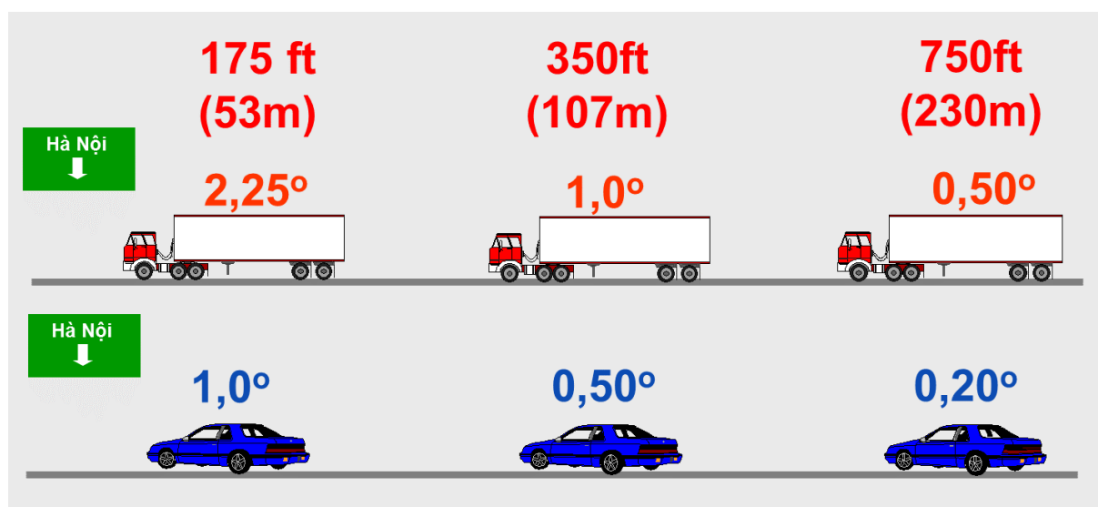
Hình E.2 (Ví dụ): Tương quan các loại xe và góc quan sát với vị trí
