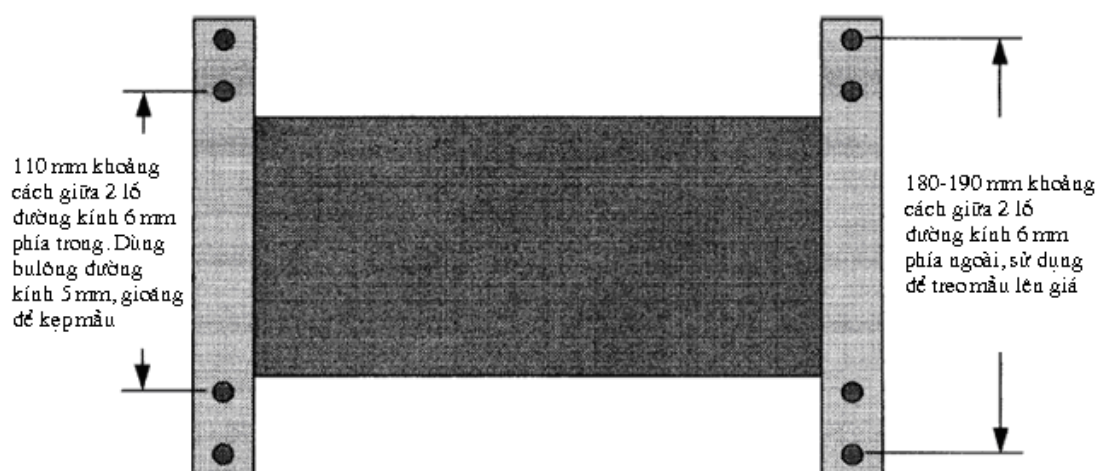
Hình 3. Sơ đồ kẹp mẫu thử nghiệm thời tiết cho màng phản quang Loại VI
